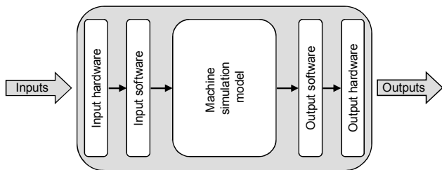
Fig. 2 HIL simulator
