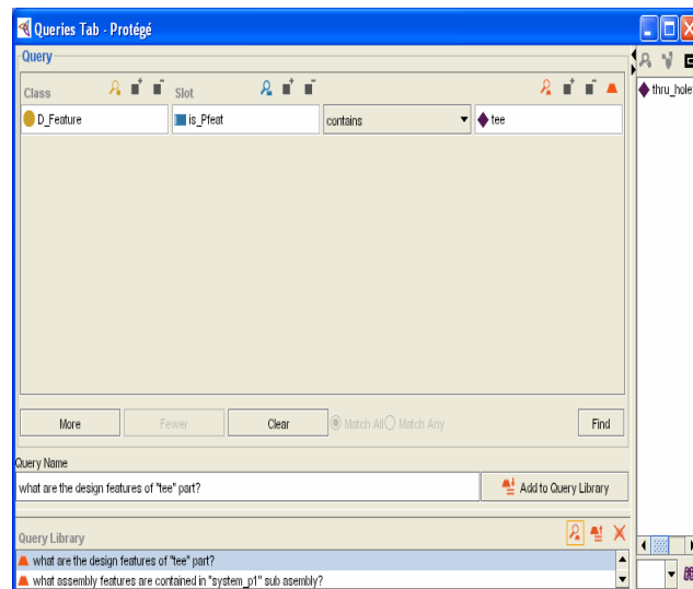
Fig. 5 Example Query
