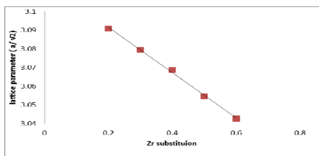
Fig. 3 Lattice parameter versus Zr substitutions
