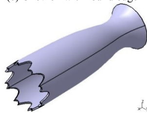
(d) Chevron with U-type edge
