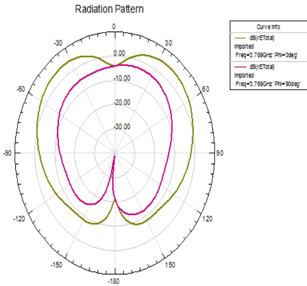
Fig. 3 (d) Simulated radiation pattern at 3.769 GHz
