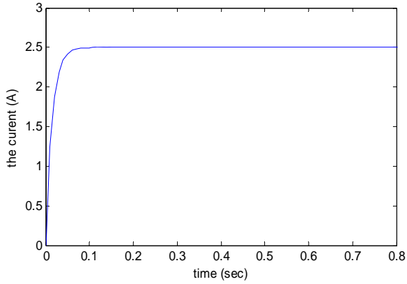
(d) Inductor current signal for line variation
