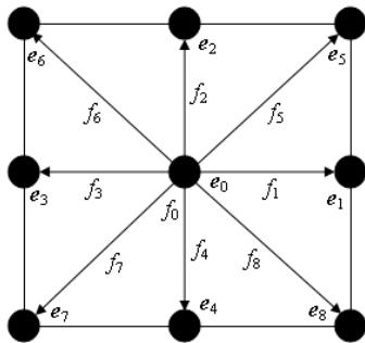
Fig. 1 D2Q9 lattice structure
