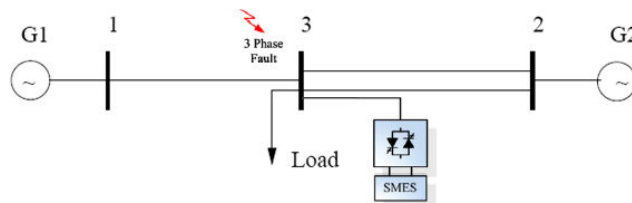
Fig. 6 IEEE 3-bus test system
