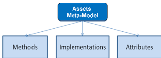
Fig. 3 Assets Meta-model
