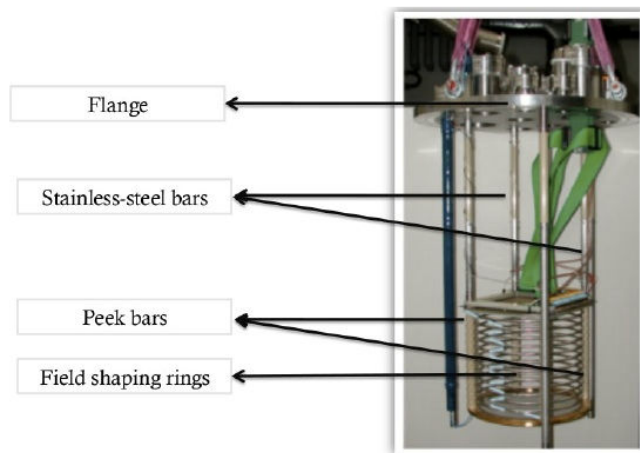
Fig. 5 LAr TPC detector
