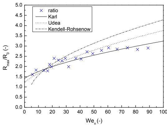
Fig. 5 R_{max}/R_0
