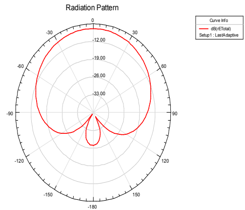
Fig. 4 (d) E-plane radiation pattern for antenna1
