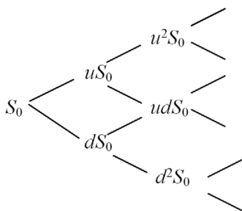
Fig. 1 Binomial tree
