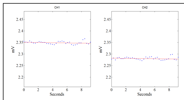
Fig. 5 RMS estimator
