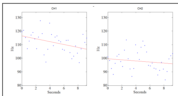
Fig. 2 MNF estimator
