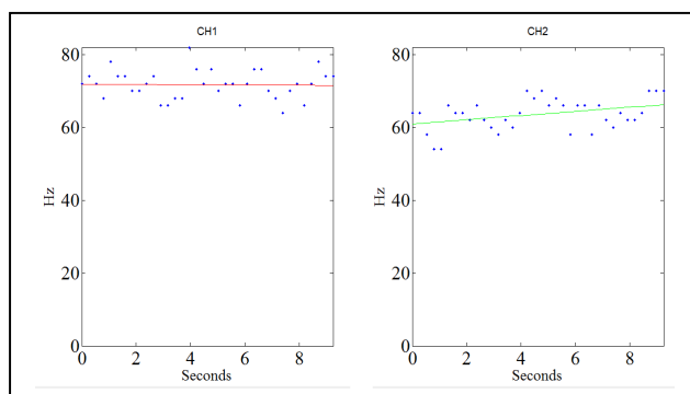
Fig. 3 MDF estimator
