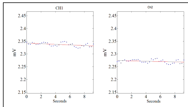
Fig. 4 ARV estimator
