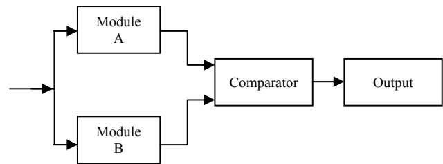
Fig. 1 Duplex module redundancy
