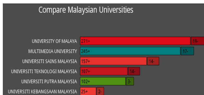
Fig. 7 OpenGL Output
