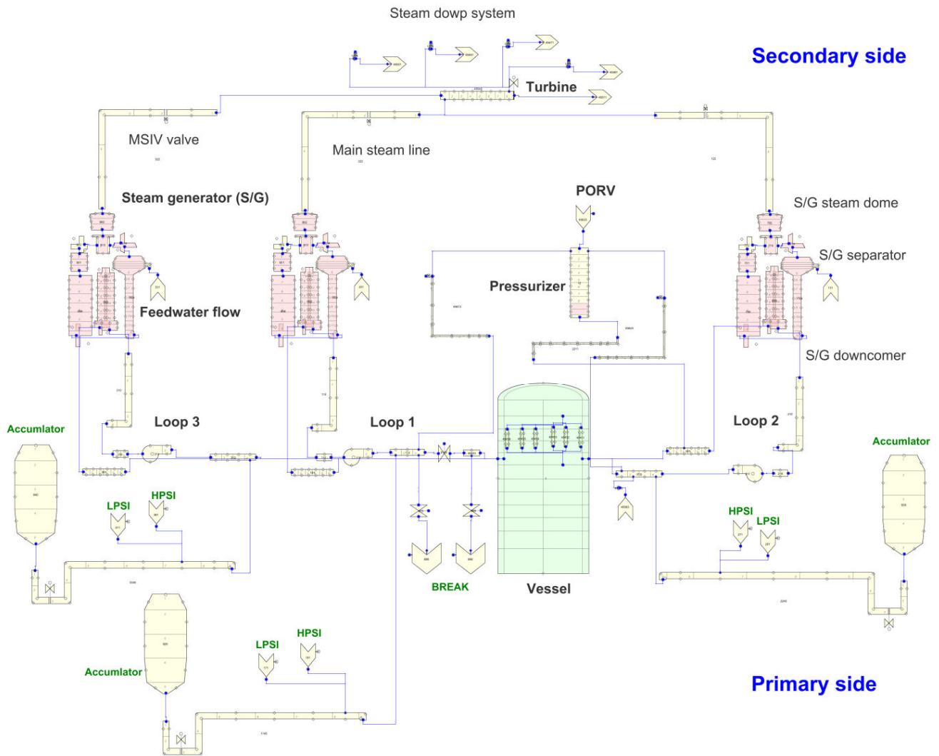
Fig. 1 Maanshan NPP TRACE model
