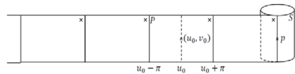
Fig. 3 The map \pi: P \rightarrow S
