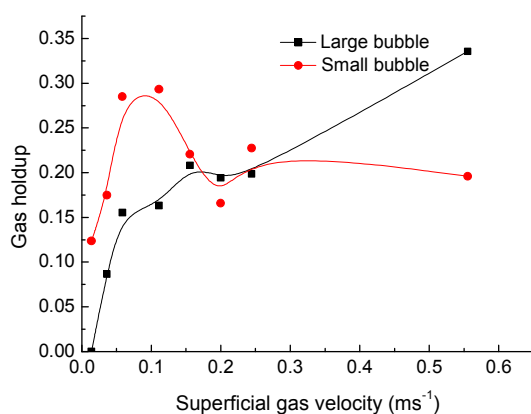
(b) 150µm
