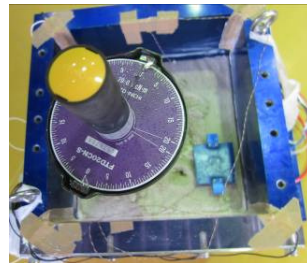
b) Vane shear test
