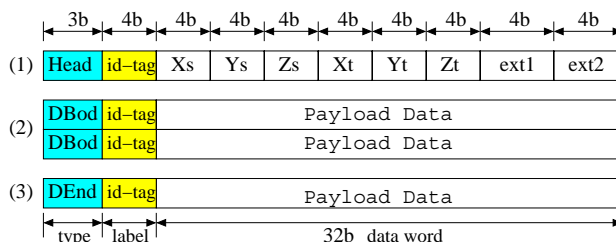
Fig. 4. Packet format.
