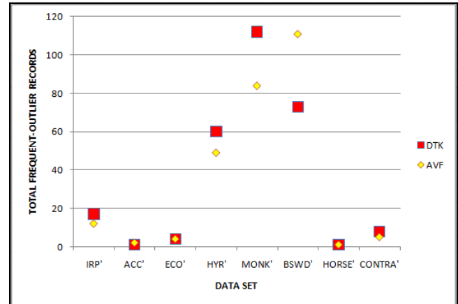
Fig. 6 DTK vs AVF
