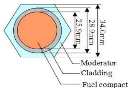
Fig. 2 Cermet MFE and cell parameters
