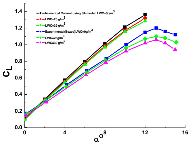
Fig. 3: CL VS AOA using SA Turbulence Model
