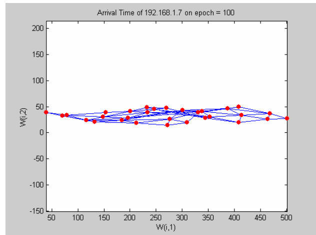
Fig. 11 Node of SOM Training on Host 4
