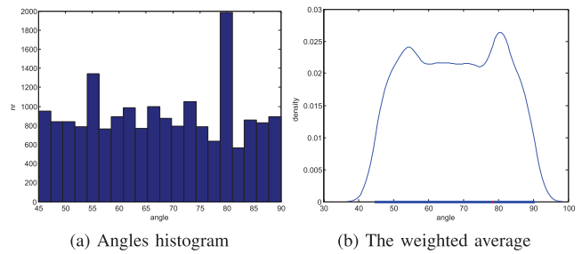
Fig. 10. Mean Shift - 1 th iteration
