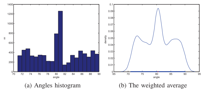
Fig. 13. Mean Shift - 4 th iteration
