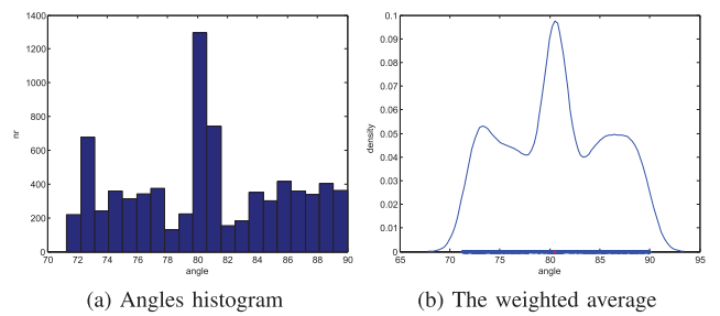
Fig. 14. Mean Shift - 5 th iteration
