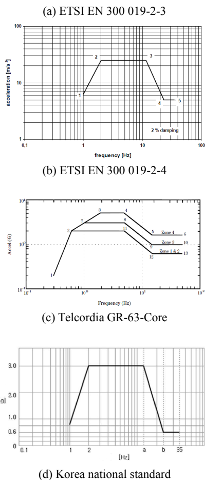
Fig. 2 Required response spectrum of each seismic standard; (a) ETSI EN 300 019-2-3, (b) ETSI EN 300 019-2-4, (c) Telcordia GR-63-Core, (d) Korea national standard
