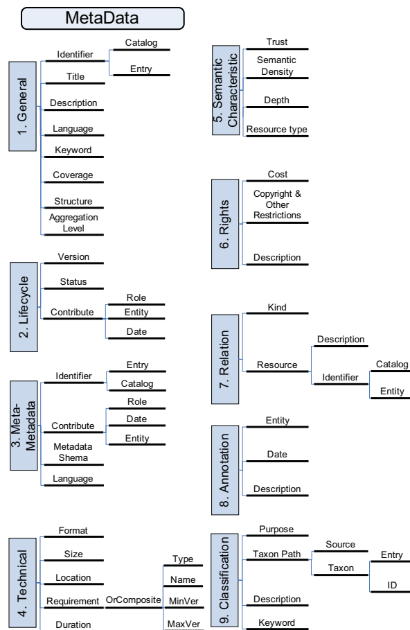
Fig. 2 Metadata Domain
