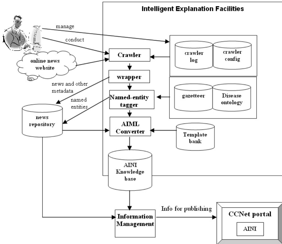
Fig. 3 AKEA Framework
