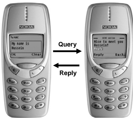
Fig. 12 SMSChat Interface
