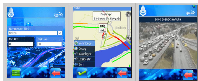
Fig. 1 IBBCepTrafik Screenshots [4].
