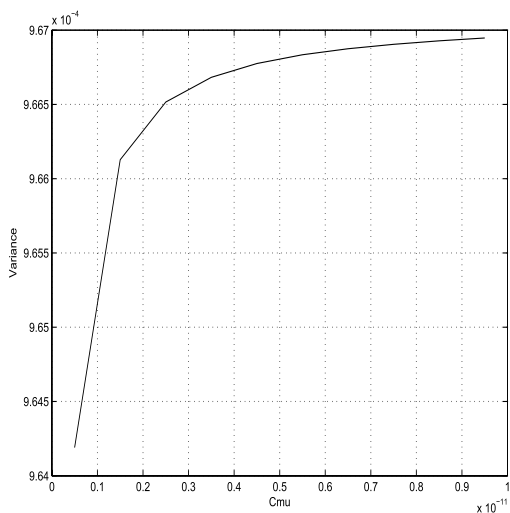
Fig. 7. Effect of device parameter C_\mu
