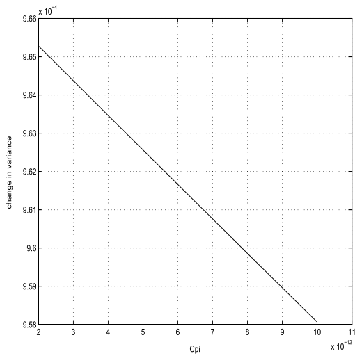
Fig. 6. Effect of device parameter C_\pi
