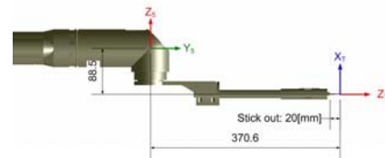
Fig. 4 Tool frame
