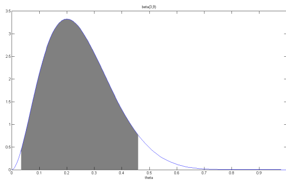
Fig. 2. LPL 0.95-credible region for a binomial parameter with \alpha=1 and \beta=1
