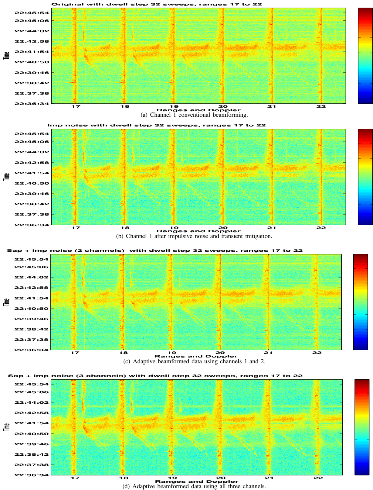
Fig. 4. Skylos OTHR data.
