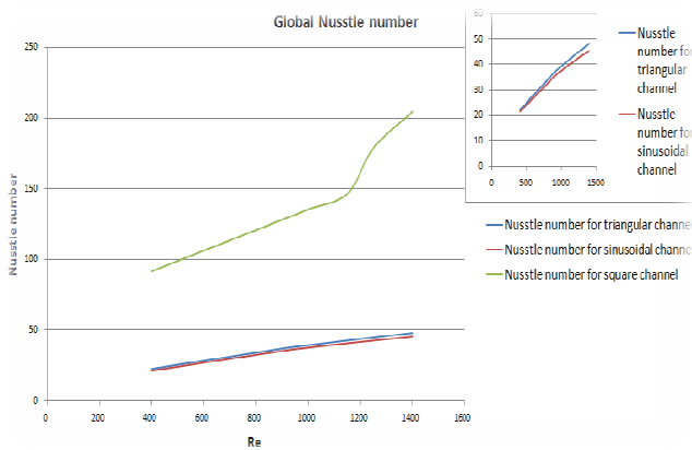
Fig. 57 Global Nusselt number
