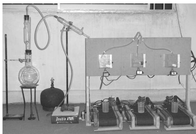
Fig. 7 Actual mechanical structure
