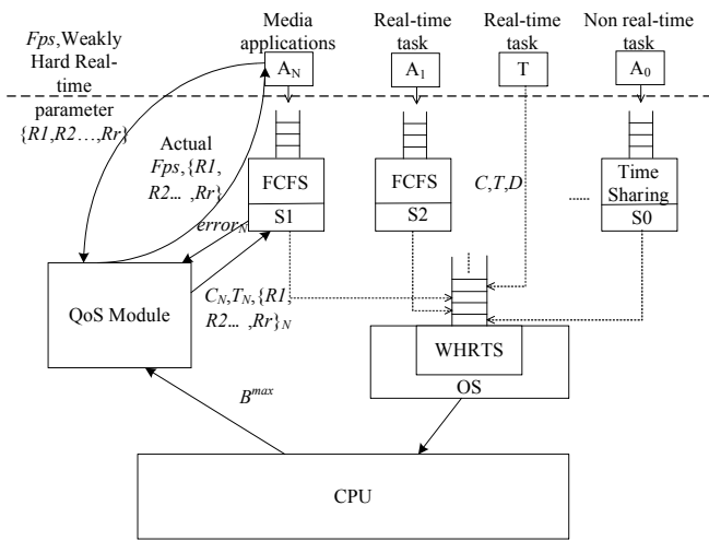
Fig. 6 QoS model
