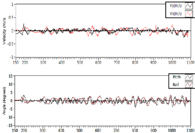
Fig. 6 AR Drone Hovering result
