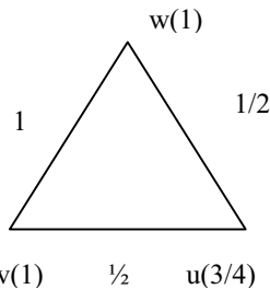
Fig. 9 G: (\sigma, \mu)
