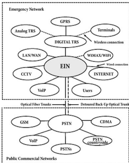
Fig. 1 Communication Architecture of EIN
