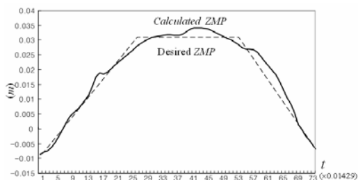
(a) ZMP trajectory
