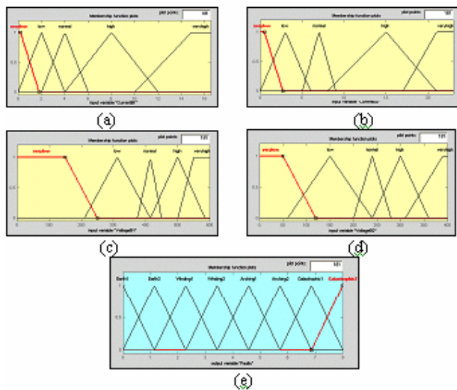
Fig. 5 Membership function for dry type transformer controller Inputs: (a) I1 (b) I2 (c) V1 (d) V2. Output: (d) Fault type
