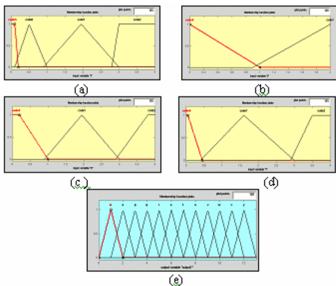
Fig. 6 Membership function for oil type transformer controller, inputs: (a) code 'i' (b) code 'j' (c) code 'k' (d) code 'l'. Output: (d) Fault type code
