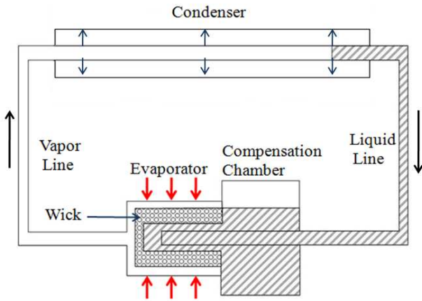
Fig. 1 LHP
