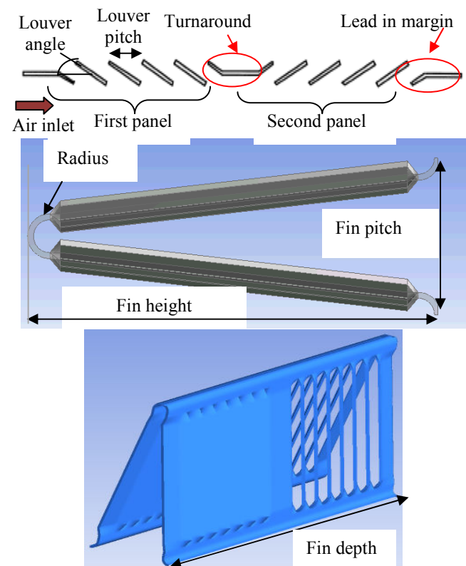
Fig. 1 Geometrical parameters of louvered fin
