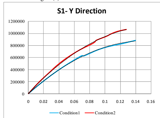
Fig. 3 (d): S1 Structure-Y direction
