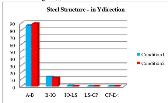
Fig. 2 (d): S1 Structure-Y direction
