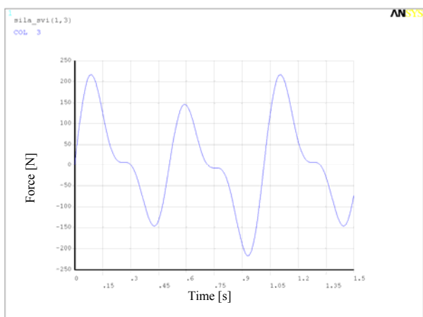
Fig. 20 Longitudal force time record
