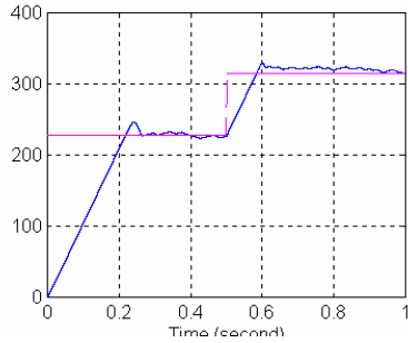
The actual motor speed
