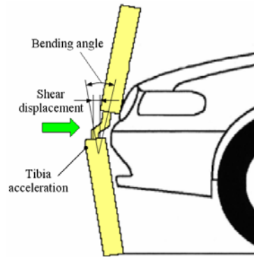
Fig. 2 Measurement parameters
