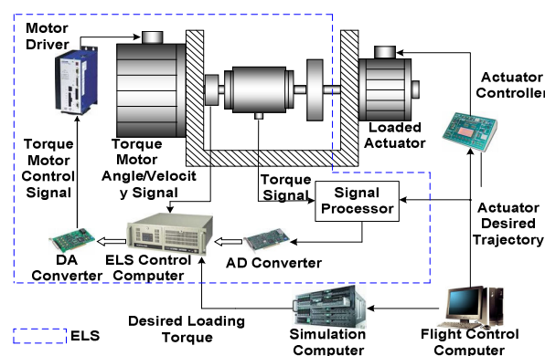
Fig. 1. Working Diagram of ELS
