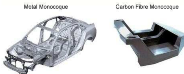
Fig. 2 Monocoque
